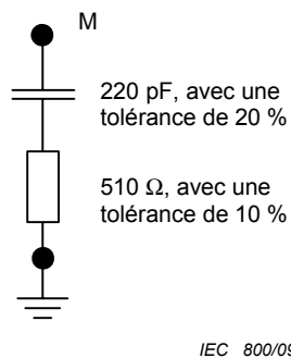
Figure 6 – Main artificielle, réseau RC (voir 7.3.5)
